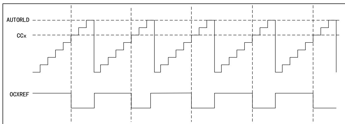
图 72 PWM1 向上计数模式的时序图
