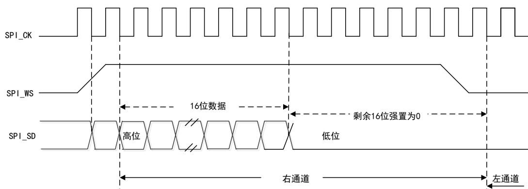
图 117 I2S 飞利浦协议波形（16 位扩展至 32 位）
