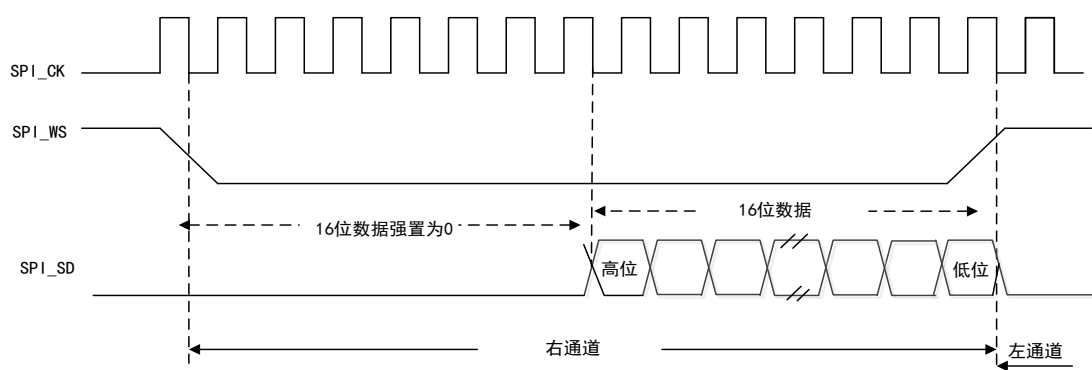
图 123 LSB 对齐标准下（16 位扩展至 32 位）
