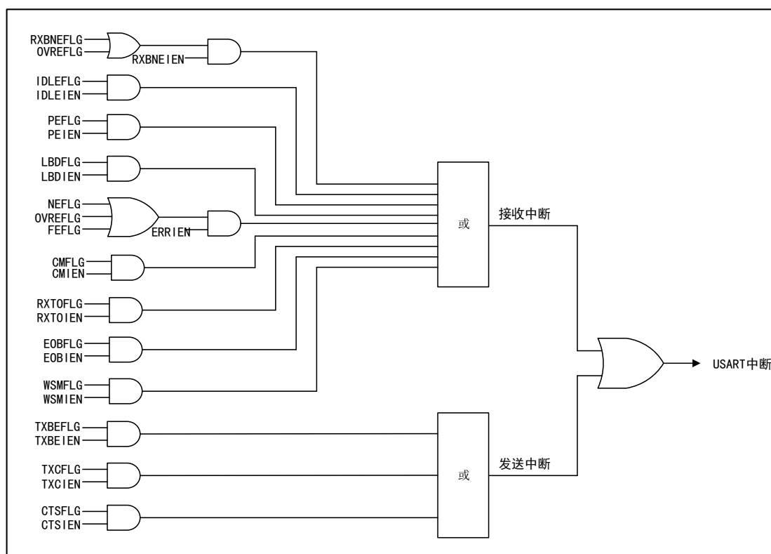
图 104 USART 中断映射
