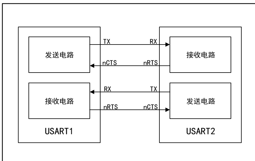
图 103 两个 USART 之间的硬件流控制
