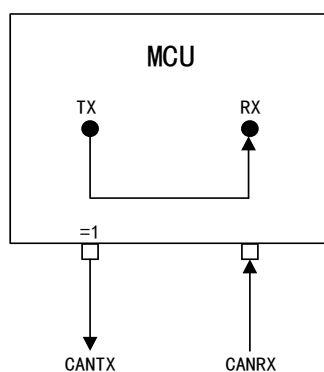
图 130 CAN 工作在静默环回模式
