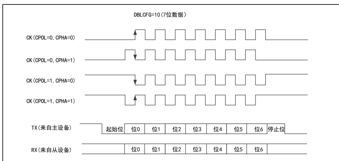
图 96 USART 同步传输时序图 (DBLCFG=10)
