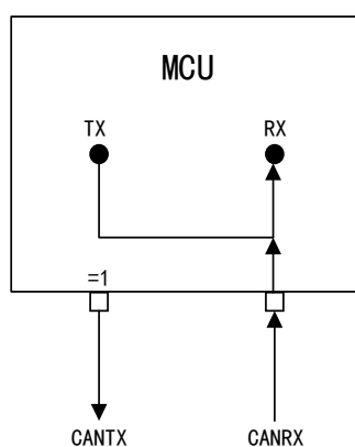
图 128 CAN 工作在静默模式
