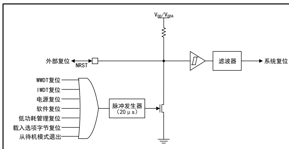
图 2 “系统复位” 复位电路
