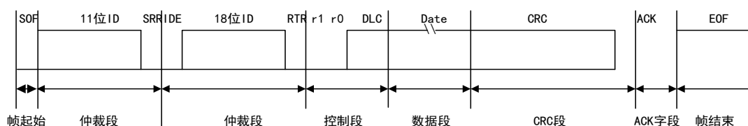
图 127 扩展数据帧
