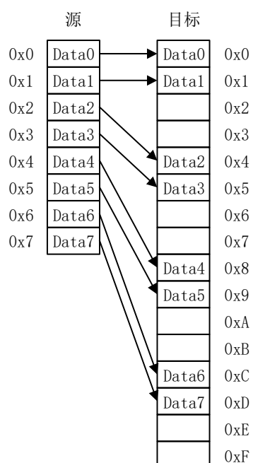
图 14 源为 16bits 目标为 32bits 的传输宽度
