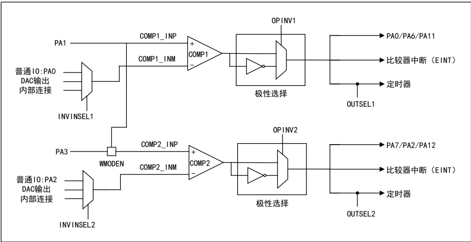
图 140 COMP 结构框图
