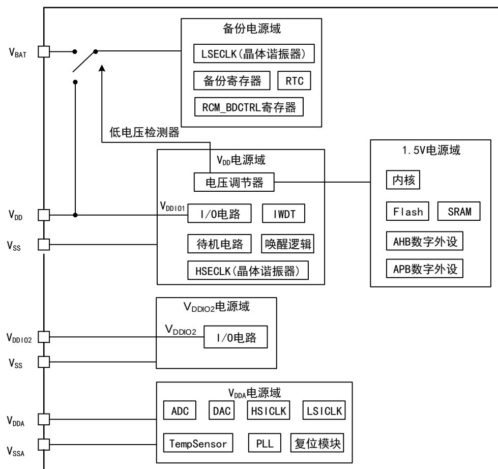
图 6 电源控制结构框图
