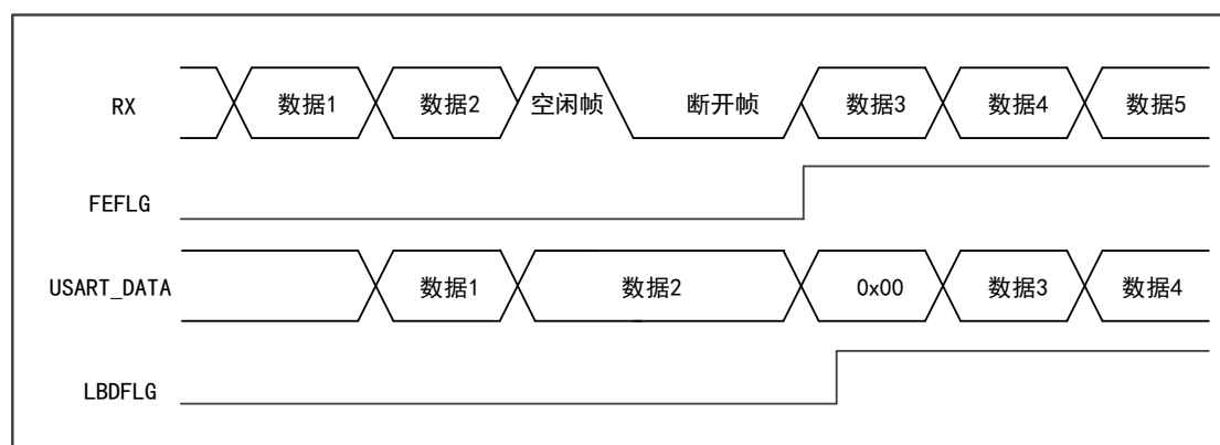
图 99 空闲状态检测断开帧
