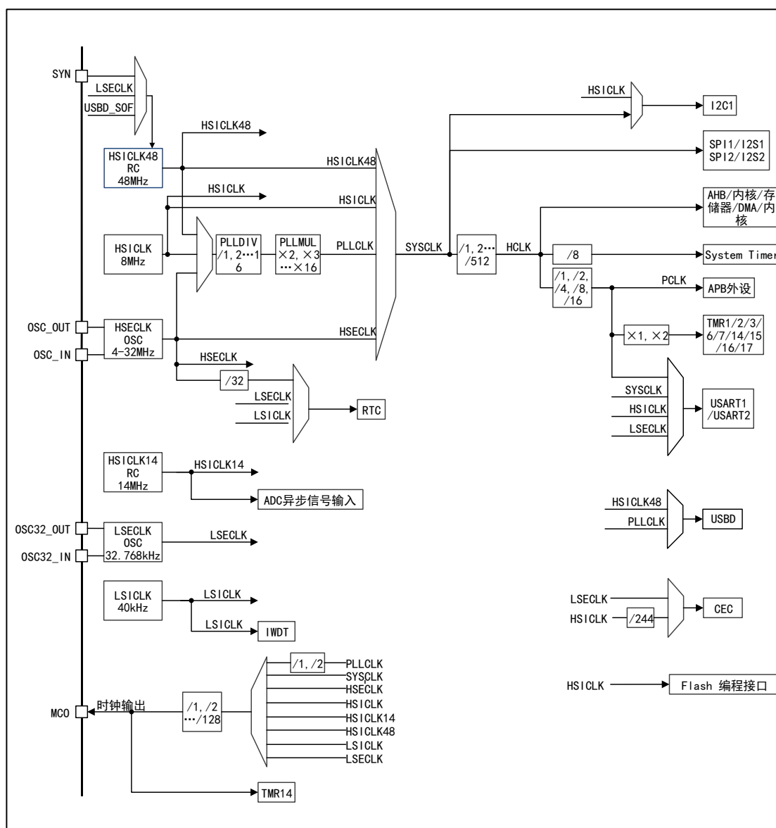
图 4APM32F072x8xB 时钟树
