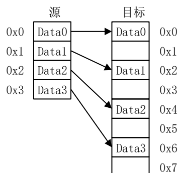
图 10 源为 8bits 目标为 16bits 的传输宽度
