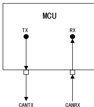
图 131 CAN 工作在正常模式
