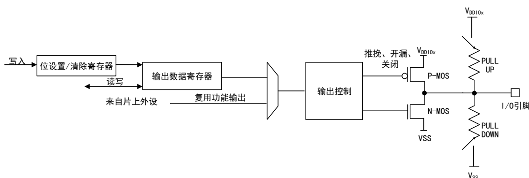
图 19 输出模式 I/O 结构
