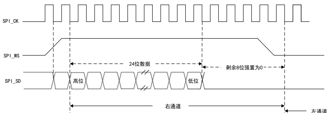
图 116 I2S 飞利浦协议波形（24 位）
