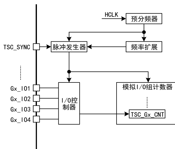
图 139 结构框图
