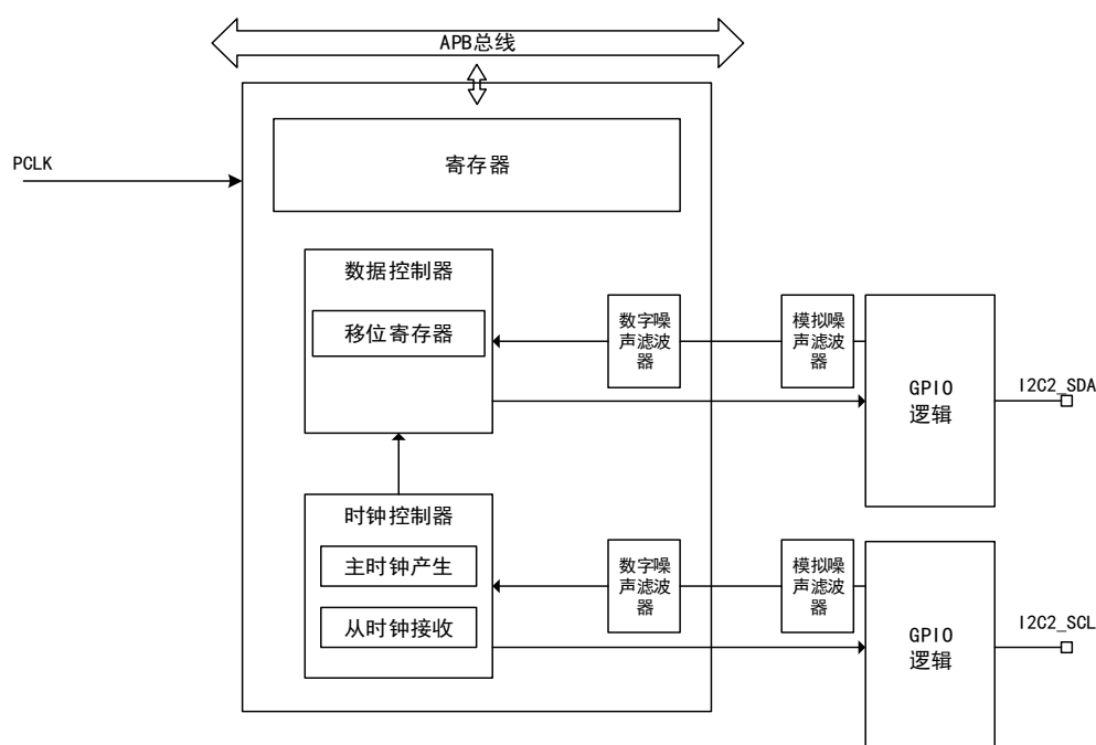
图 106 I2C2 功能结构图
