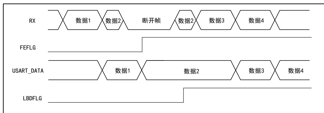
图 100 数据传输状态检测断开帧
