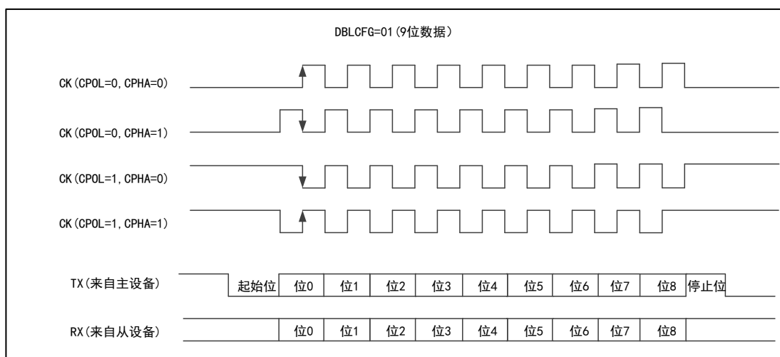
图 98 USART 同步传输时序图 (DBLCFG=01)
