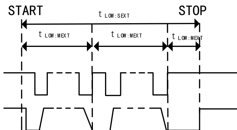
图 110 t_{\text{LOW:SEXT}} 与 t_{\text{LOW:MEXT}} 时间
